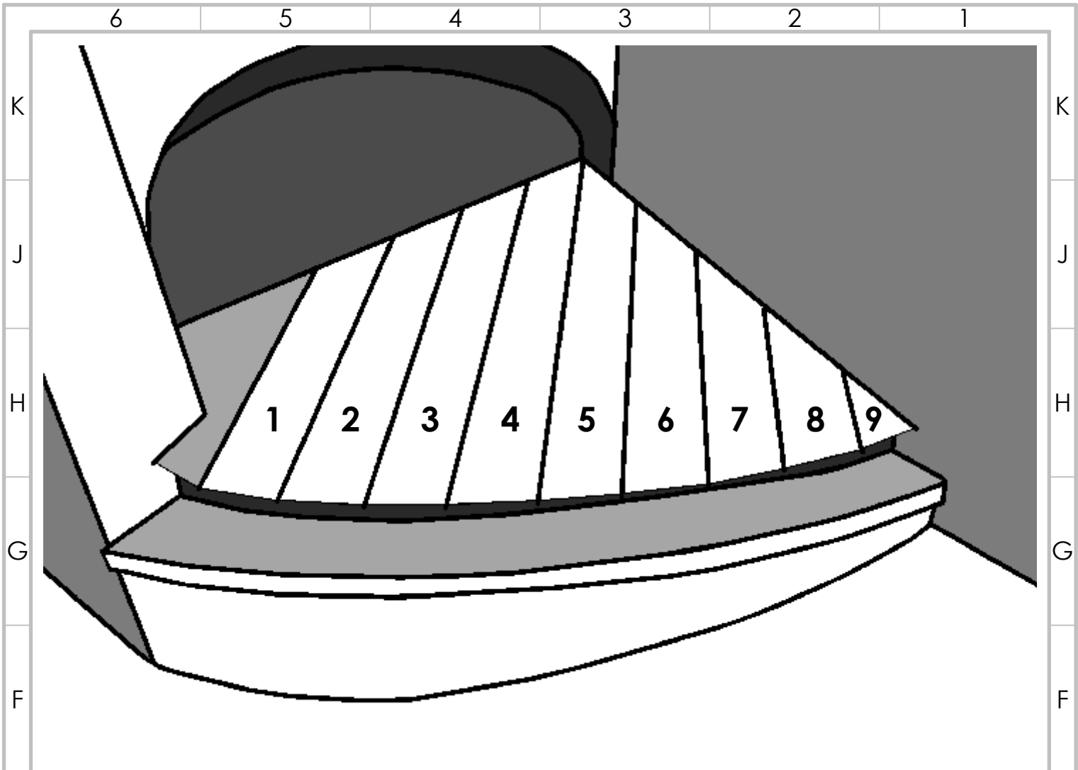
Vue d'ensemble de la verrière depuis l'exterieur. 9 pièces en verre Feuilleté 44.2 (8.8 mm) Opale.
